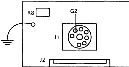
S26381-D226-V1 (Bauteileseite)
