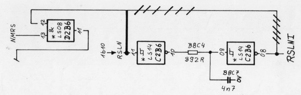
Ausschnitt aus Schaltplan 5112 291 75600-130 Blatt 5
