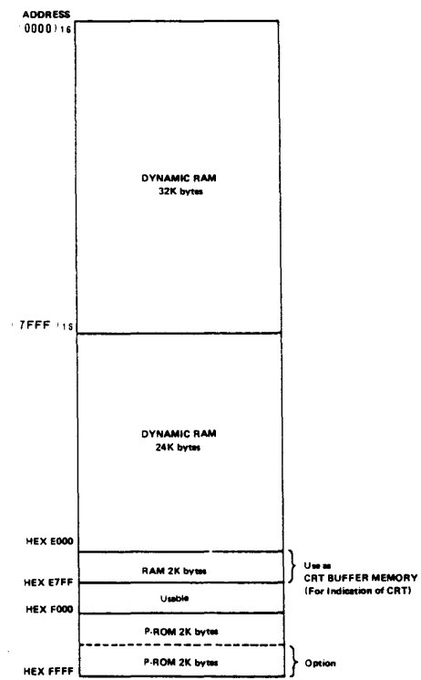
Fig. 2 - 15 MEMORY MAP
