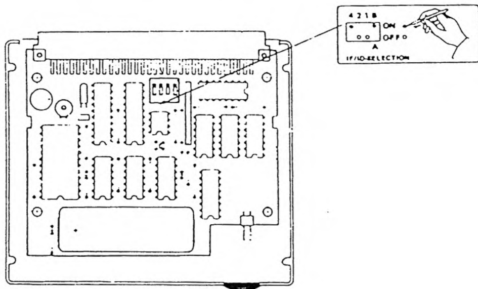
Abbildung 1.2 IFSEL-Schalter
