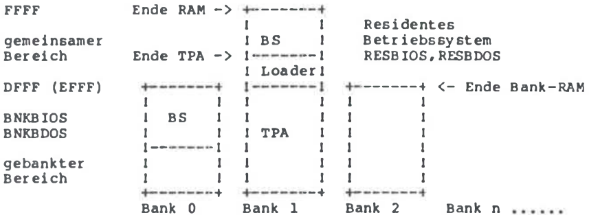
Bild 1. logische Speicheraufteilung unter CP/M 3
